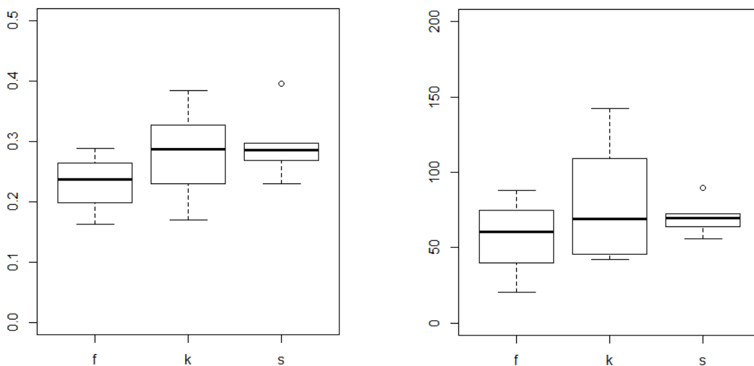
Obr. 15 Výsledky testování odolnosti glochidií škeblice proti modelovým antiparazitním koupelím (f: formaldehyd - \text{CH}_2\text{O} , k: kontrolní skupina, s: chlorid sodný – NaCl). Zobrazena je úspěšnost metamorfózy glochidií (podíl na celkovém počtu přichycených) (vlevo) a celkový počet úspěšně vyvinutých juvenilních jedinců (vpravo) na jednotlivých rybách.
